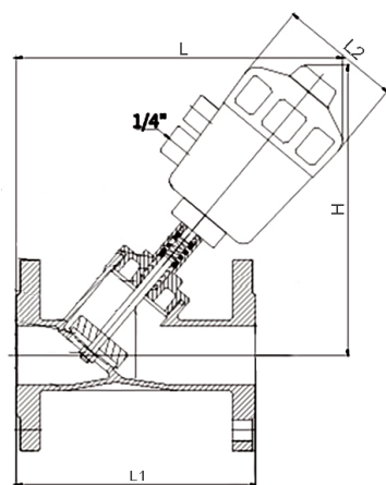
外形简图
