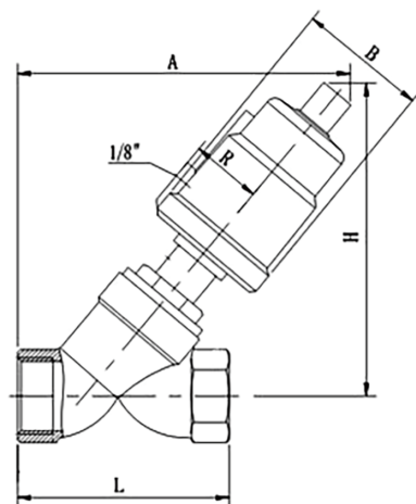
外形简图
