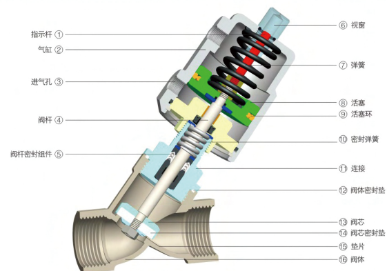
外形剖面图
