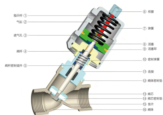
外形剖面图
