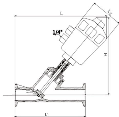
外形简图
