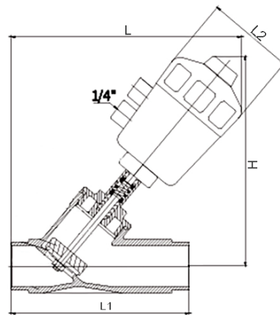
外形简图
