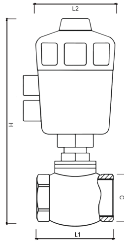
外形简图
