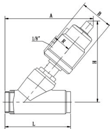
外形简图
