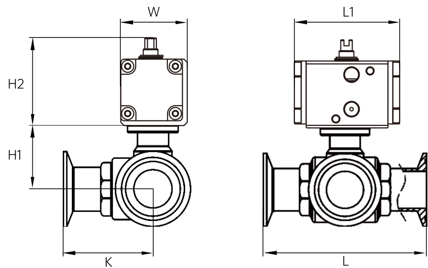
外形简图
