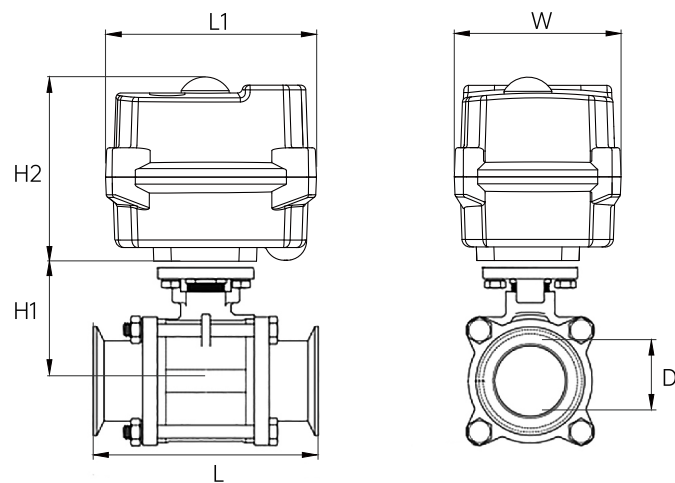
外形简图
