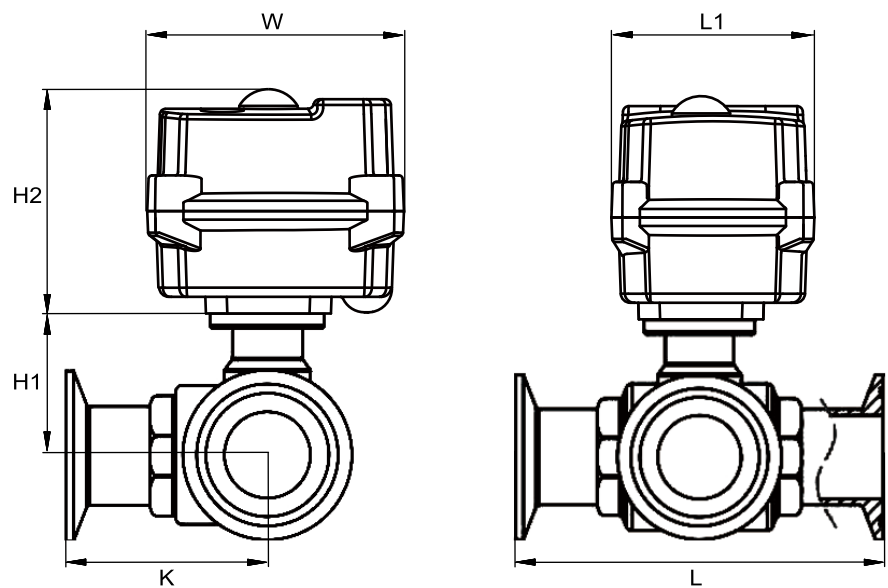
外形简图
