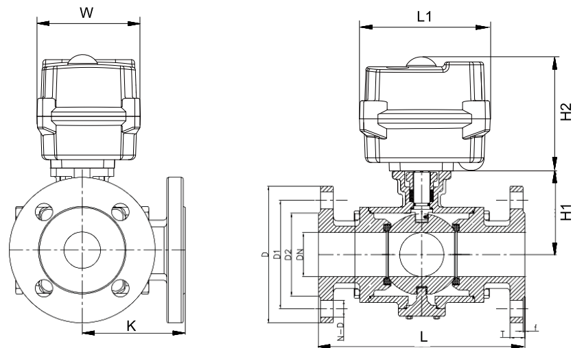
外形简图
